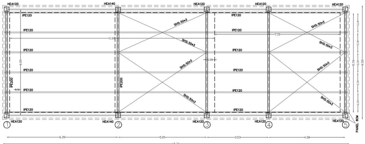
ΣΥΛΟΤΥΠΟΣ ΣΤΕΓΗΣ
