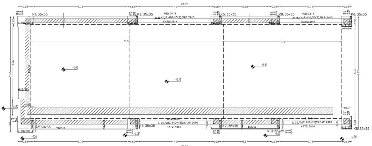
ΣΥΛΟΤΥΠΟΣ ΘΕΜΕΛΙΩΣΗΣ
